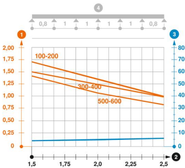
Діаграма навантаження, кабельний лоток типу MKSM 85
